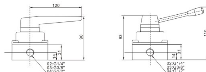
铁手柄时主视图
